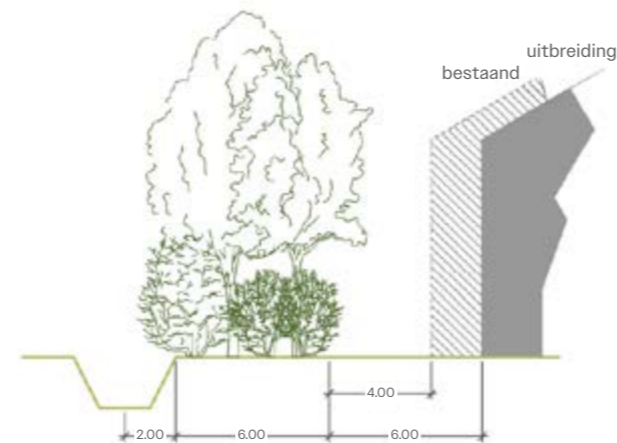
Figuur 8: Maatvoering erfsingels
